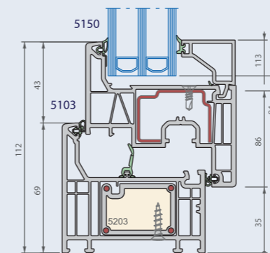
Sección vertical
