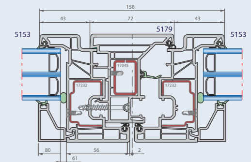
Sección horizontal
