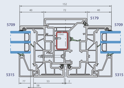
Sección horizontal
