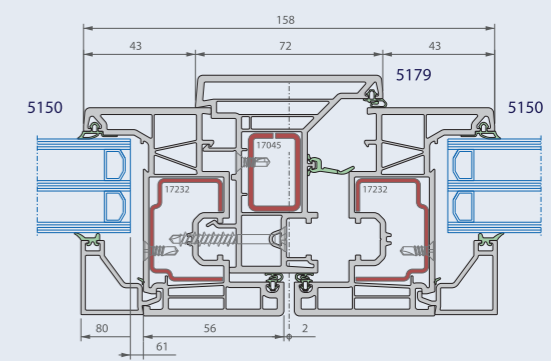
Sección horizontal
