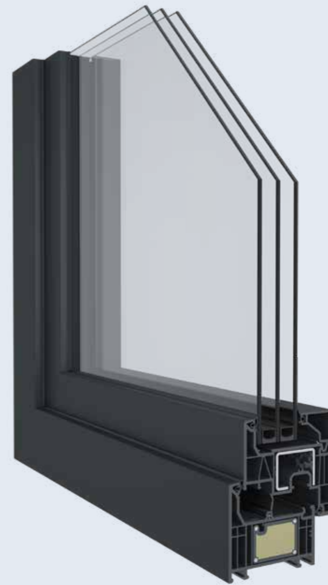
Sección vertical
