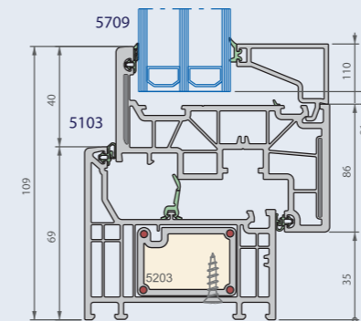
Sección vertical
