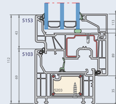
Sección vertical
