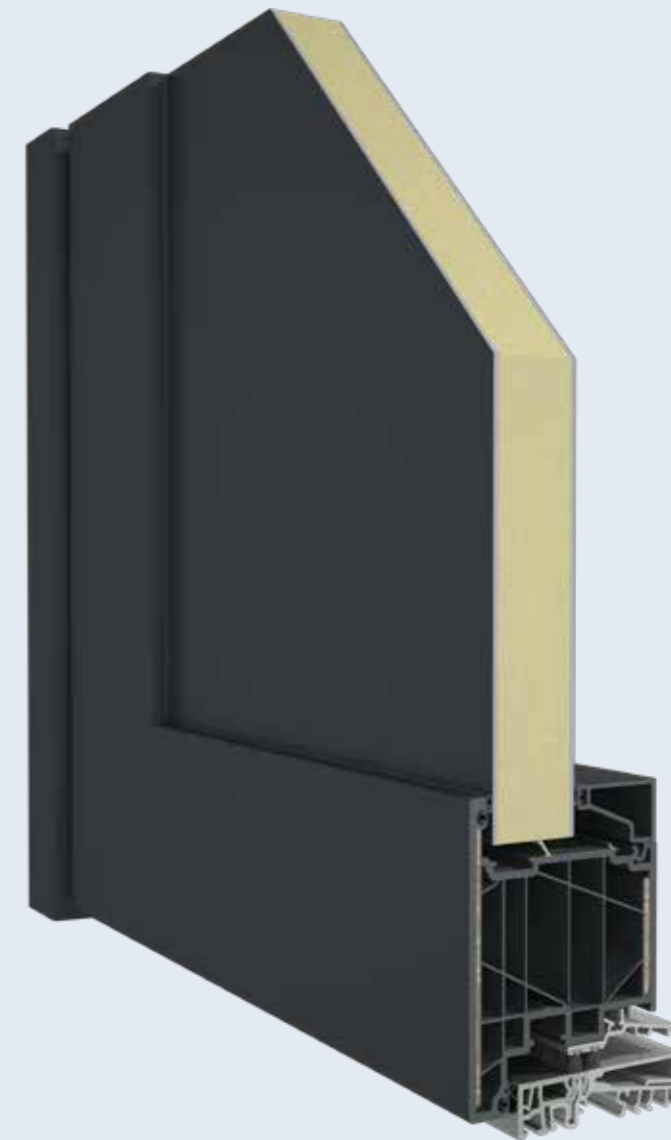
Sección vertical
