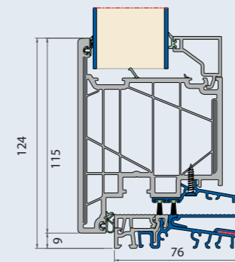
Sección vertical
